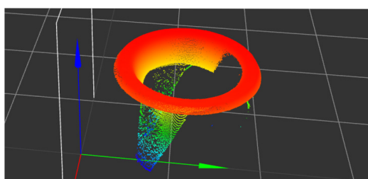
3D модель конусообразного отверстия, монокулярный сканер
