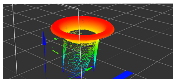
3D модель конусообразного отверстия, бинокулярный сканер
